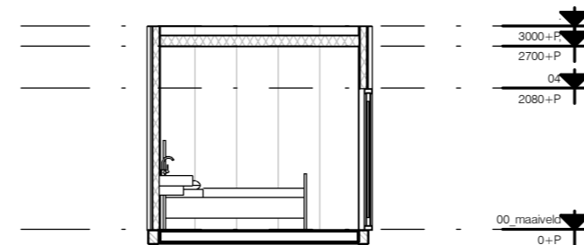
doorsnede 01
